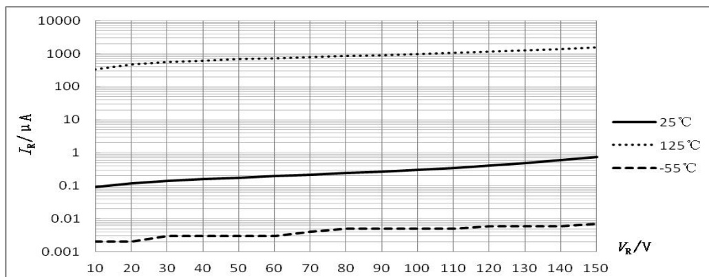
图1 I_R — V_R 特性曲线
