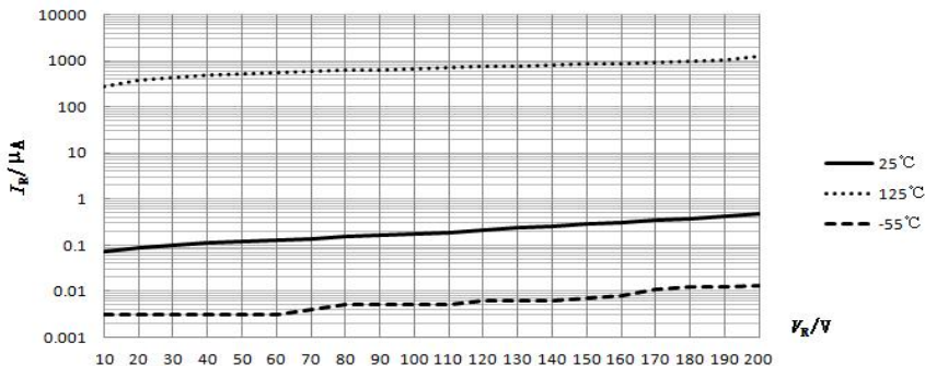
图 1 I_R-V_R 特性曲线
