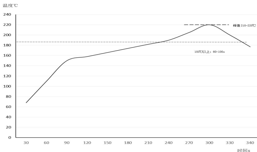
图 8 建议的回流焊曲线
