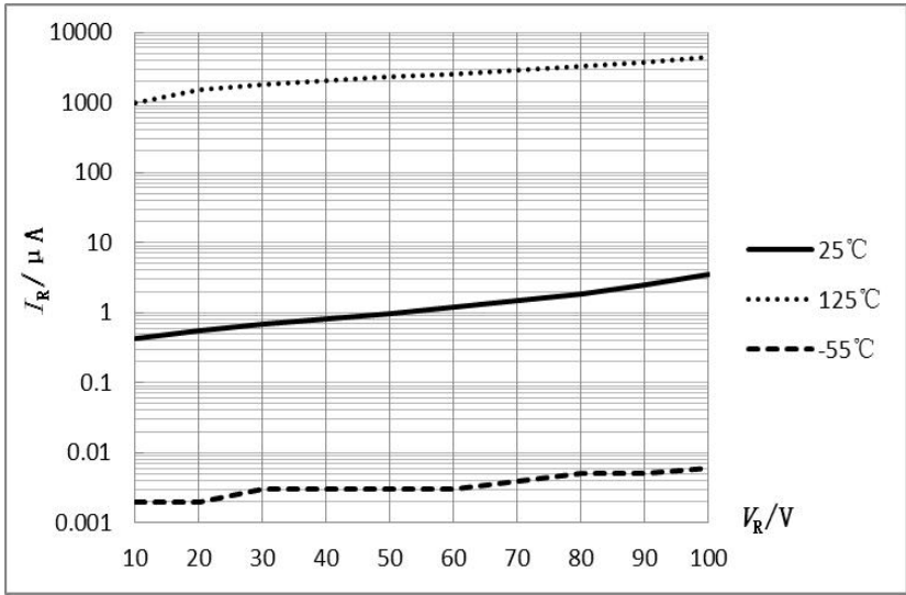
图 1 I_R-V_R 特性曲线
