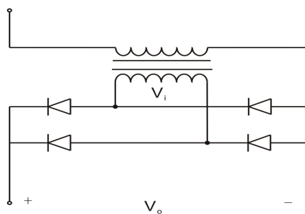
图 6 单相全波整流电路
