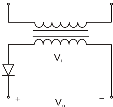
图 5 单相半波整流电路
