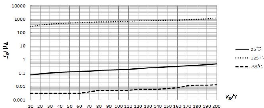
图 1 I_R-V_R 特性曲线
