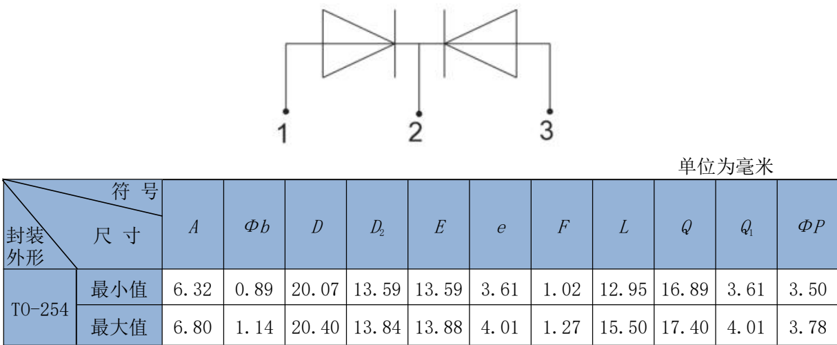
图 3 T0-254 外形尺寸
