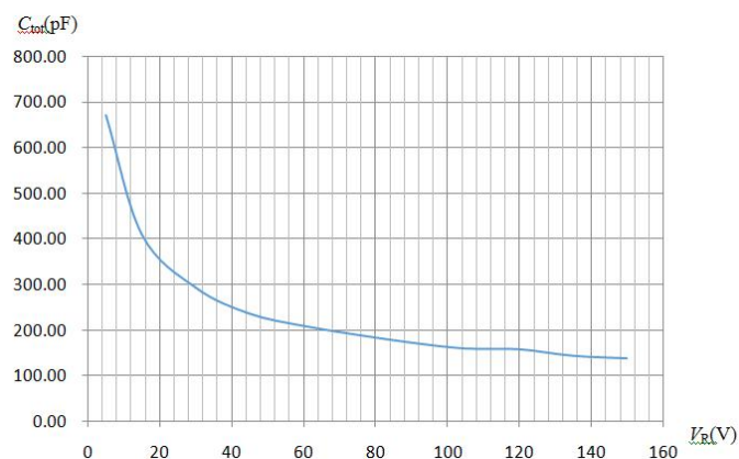
图 3 C_{tot} — V_R 特性曲线
