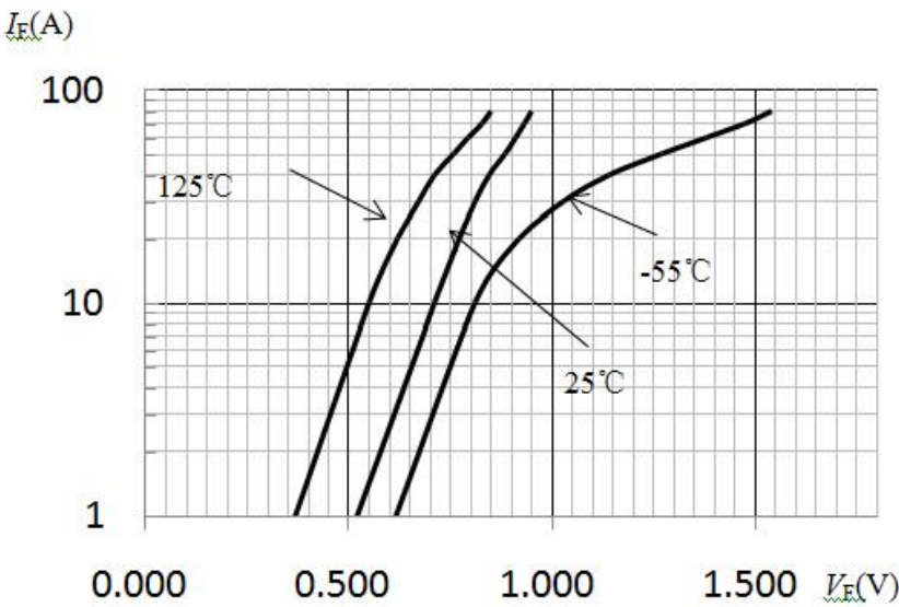
图 2 V_F-I_F 特性曲线
