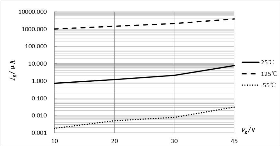
图 1 I_R-V_R 特性曲线
