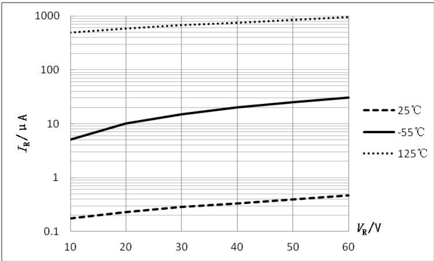
图 1 I_{\text{R}}-V_{\text{R}} 特性曲线
