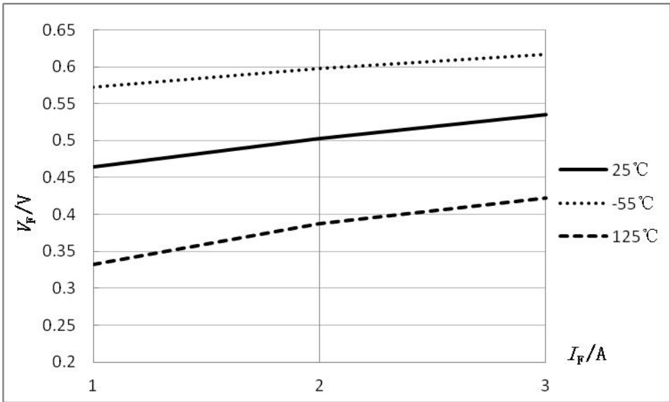
图 2 V_{\text{F}}-I_{\text{F}} 特性曲线
