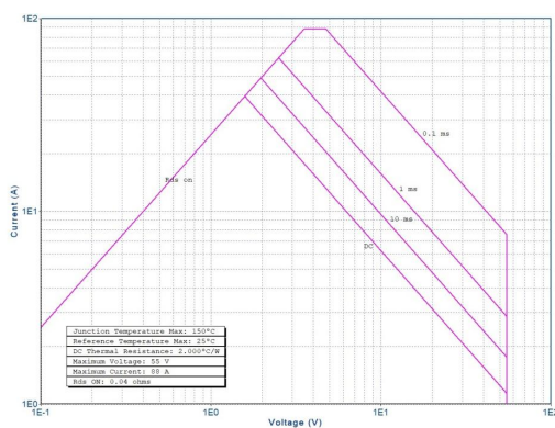
图 6 安全工作区曲线
