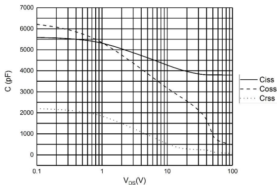
图 4 电容曲线
