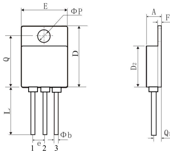
图 7 SMD-0.2、SMD-0.5 型封装外形尺寸
