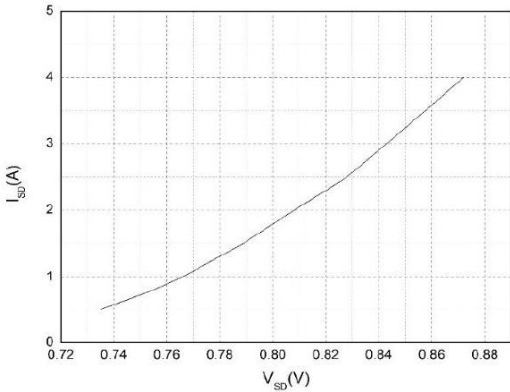
图 2 体二极管特性曲线
