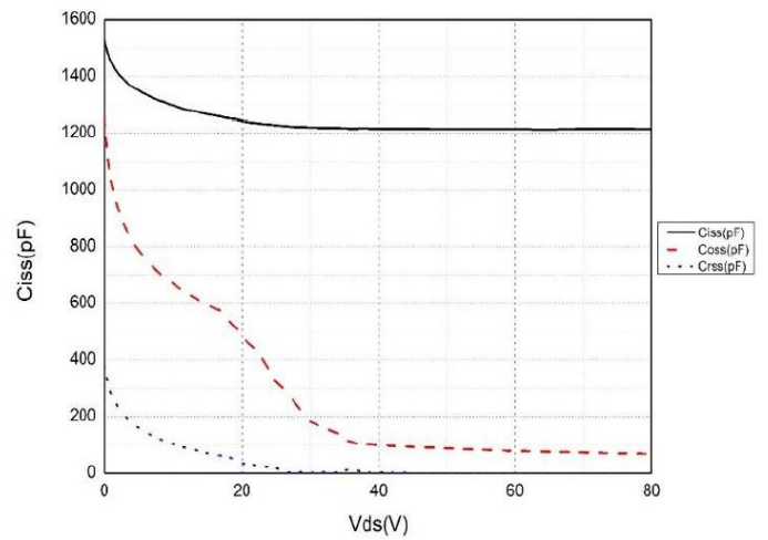
图 4 电容曲线
