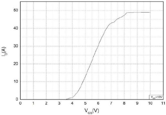
图 1 转移特性曲线
