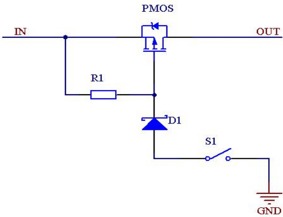
图 7 典型开关电路
