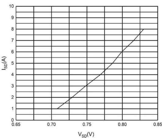
图 2 体二极管特性曲线
