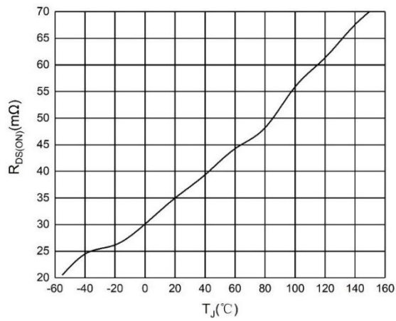
图 3 R_{DS(on)}-T_J 特性曲线
