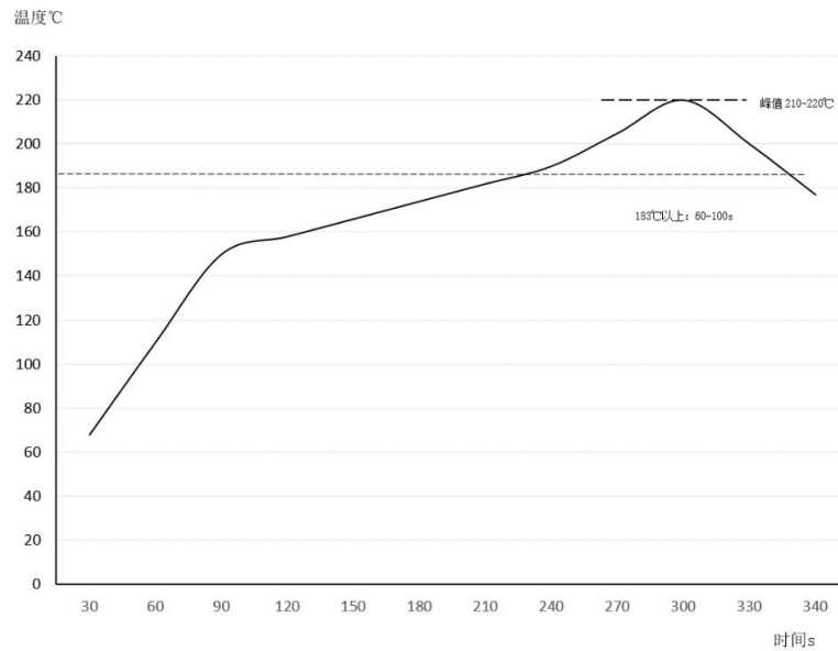
图 10 建议的回流焊曲线
