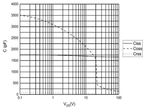
图 4 电容曲线
