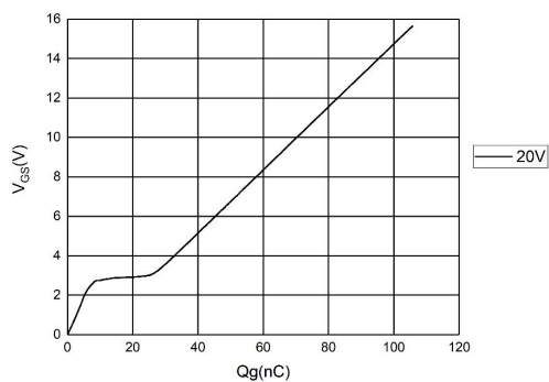
图 5 V_{GS}-Q_g 特性曲线
