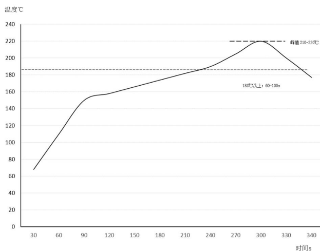
图 11 建议的回流焊曲线
