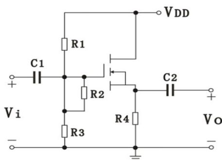
图 10 共漏极放大电路
