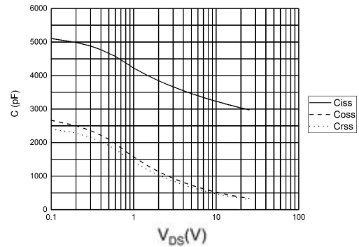
图 4 电容曲线
