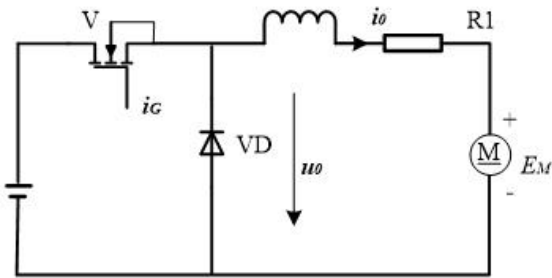
图 9 典型开关电路
