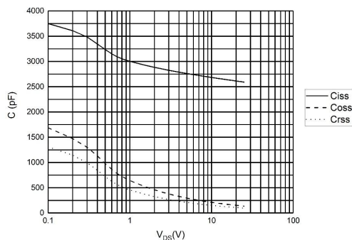
图 4 电容曲线
