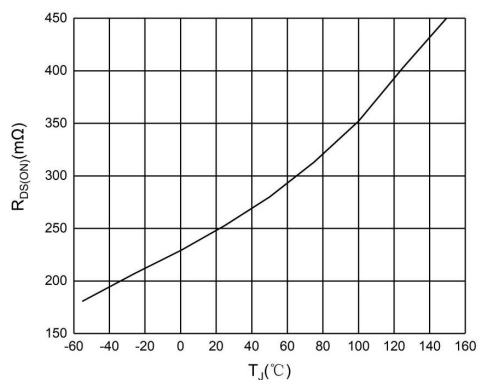
图 3 R_{DS(on)}-T_J 特性曲线
