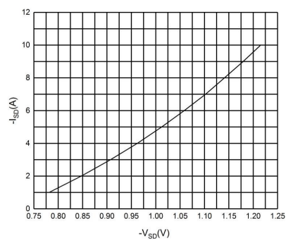
图 2 体二极管特性曲线
