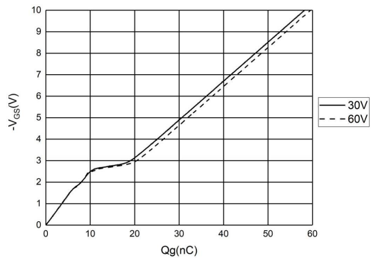
图 5 特性曲线
