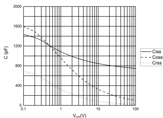
图 4 电容曲线
