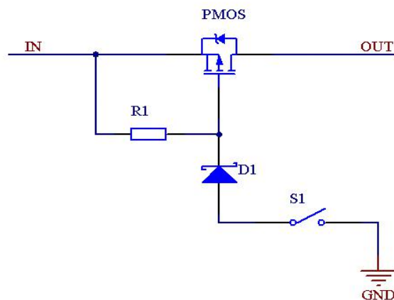
图 8 典型开关电路
