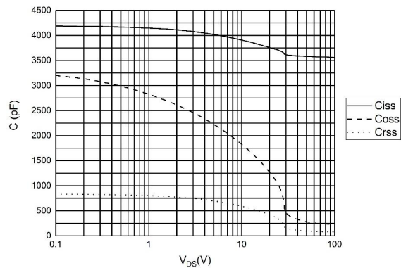
图 4 电容曲线
