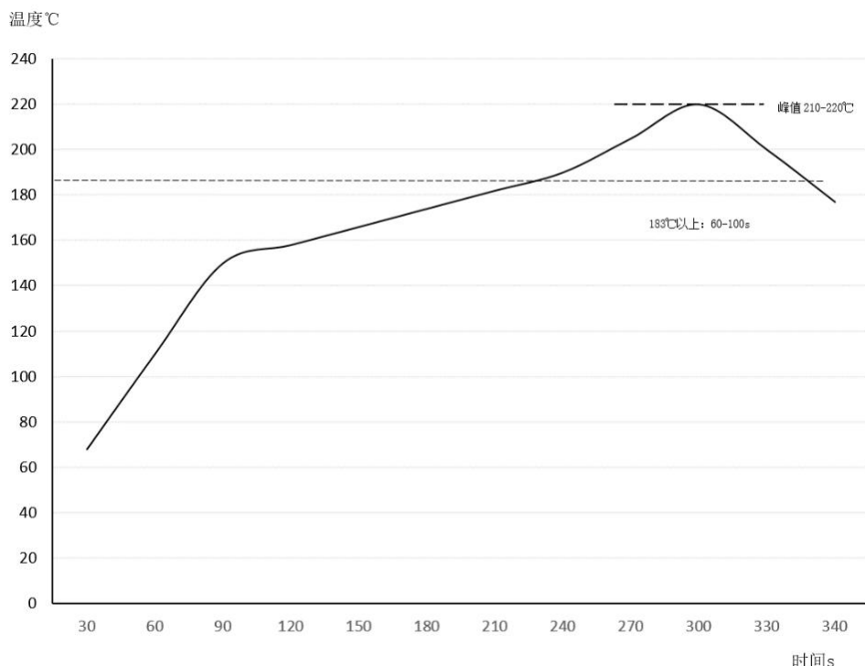
图 11 建议的回流焊曲线
