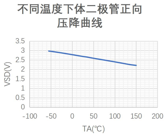
图 3 体二极管正向压降特性曲线
