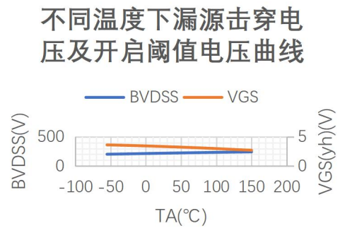
图 2 漏源击穿电压、阈值电压特性曲线
