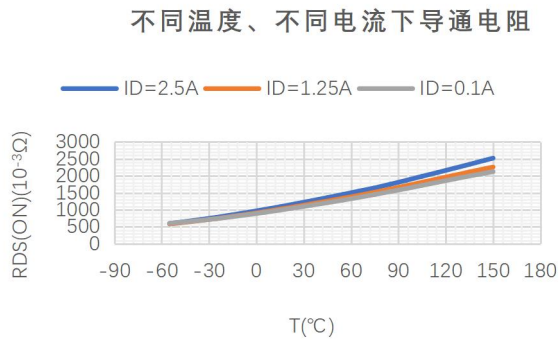
图 1 导通电阻特性曲线
