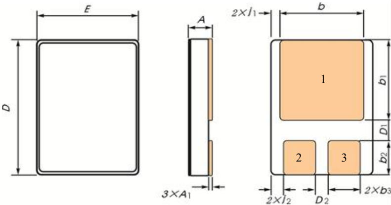
图 4 T0-257 外形尺寸
