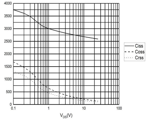
图 4 电容曲线
