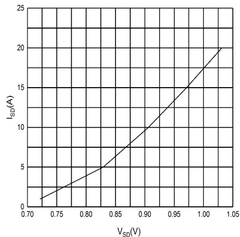
图 2 体二极管特性曲线
