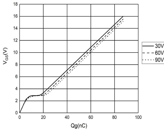
图 5 V_{GS}-Q_g 特性曲线
