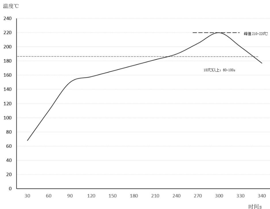
图 11 建议的回流焊曲线
