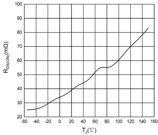
图 3 R_{DS(on)}-T_J 特性曲线
