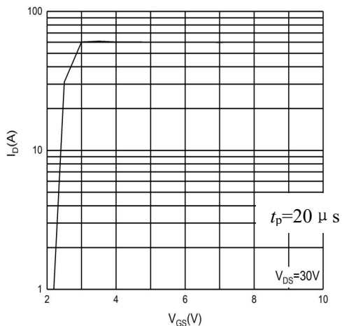
图 1 转移特性曲线
