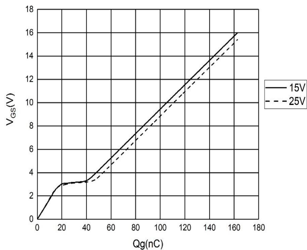
7.5 I_D=12A 时, 不同 V_{DS} 下, Q_g 随 V_{GS} 的变化曲线
