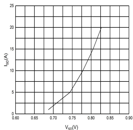
图 2 体二极管特性曲线
