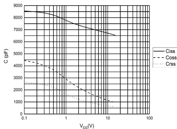
7.4 V_{GS}=0V , f=1MHz 时, 电容 C 随 V_{DS} 的变化曲线
