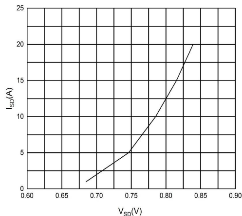
图 2 体二极管特性曲线
