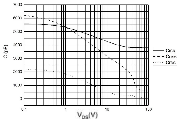
图 4 电容曲线
