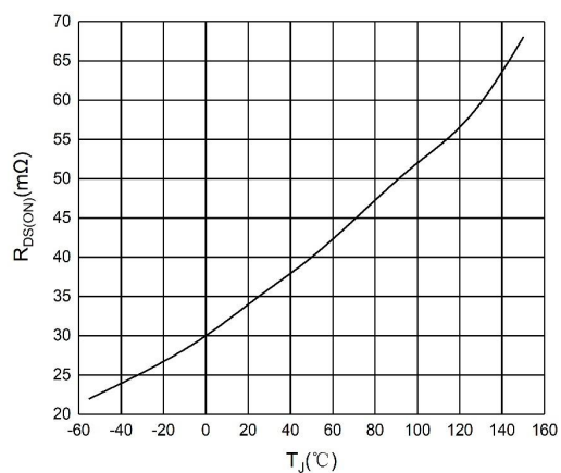
图 3 R_{DS(on)}-T_J 特性曲线
