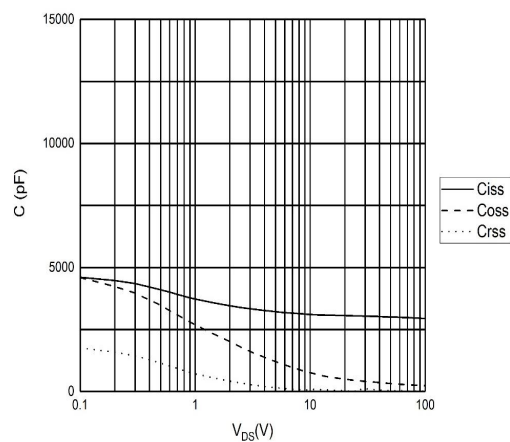
图 4 电容曲线
