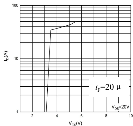
图 1 转移特性曲线
