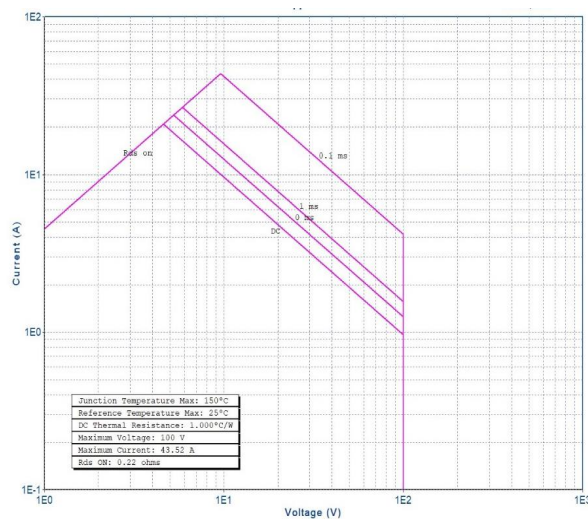
图 6 安全工作区曲线
