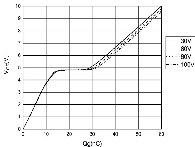
7.5 I_D=18A 时, 不同 V_{DS} 下, Q_g 随 V_{GS} 的变化曲线
