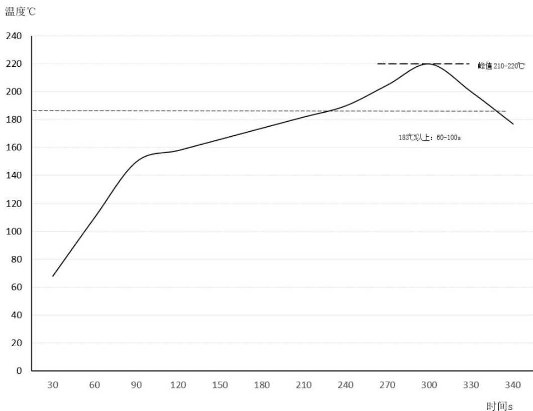
图 11 建议的回流焊曲线
