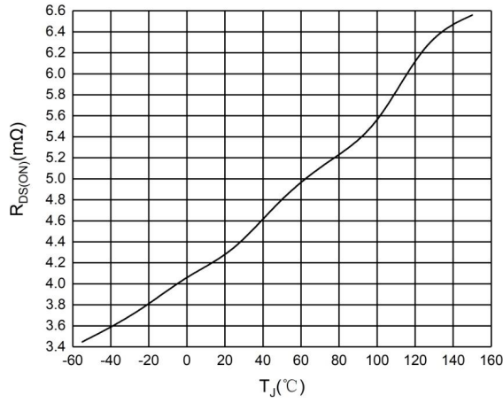
图 3 R_{DS(on)}-T_J 特性曲线
