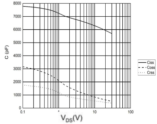
7.4 V_{GS}=0V , f=1MHz 时, 电容 C 随 V_{DS} 的变化曲线
