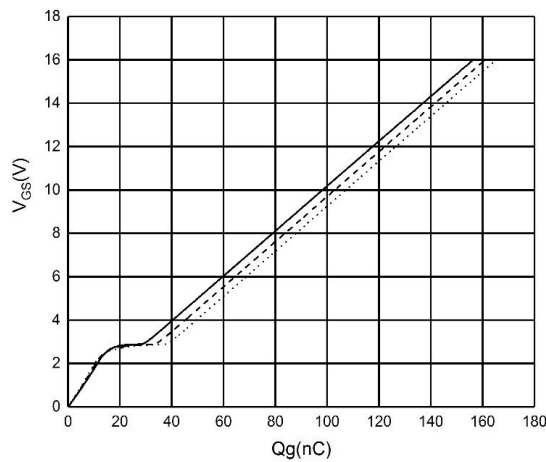
图 5 V_{GS}-Q_g 特性曲线
