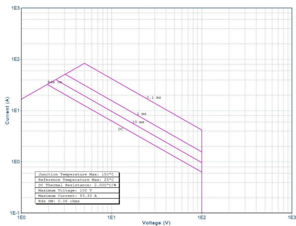
图 5 安全工作区曲线
