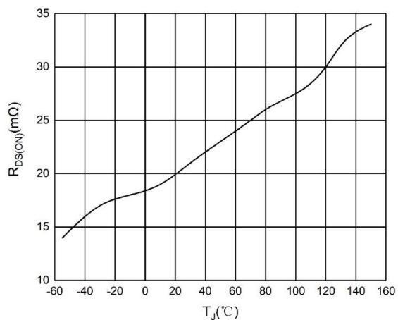
图 1 R_{DS(on)} - T_J 特性曲线
