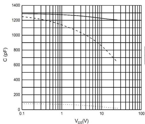
图 3 电容曲线
