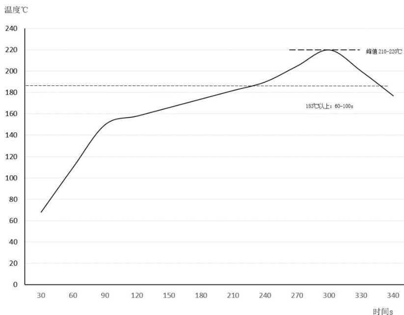
图 10 建议的回流焊曲线
