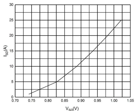
图 2 体二极管特性曲线
