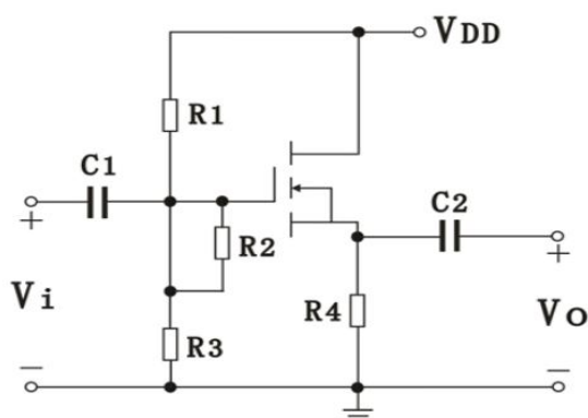
图 10 共漏极放大电路
