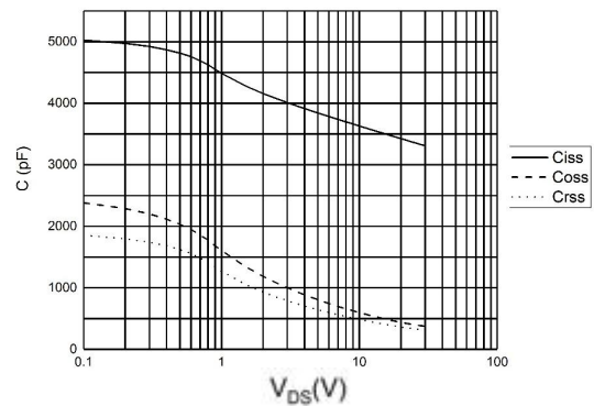
图 4 电容曲线
