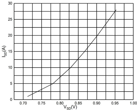
图 2 体二极管特性曲线
