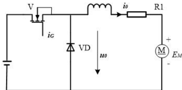
图 9 典型开关电路
