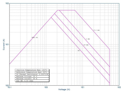
图 6 安全工作区曲线
