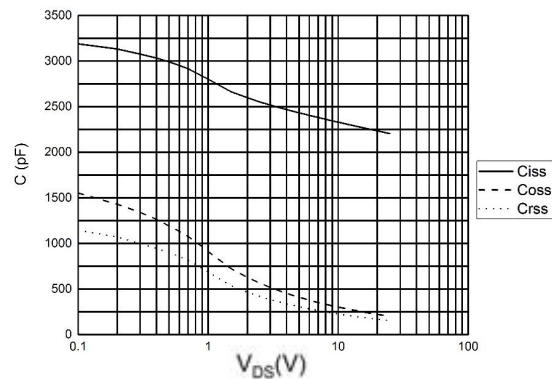
图 4 电容曲线
