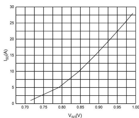
图 2 体二极管特性曲线
