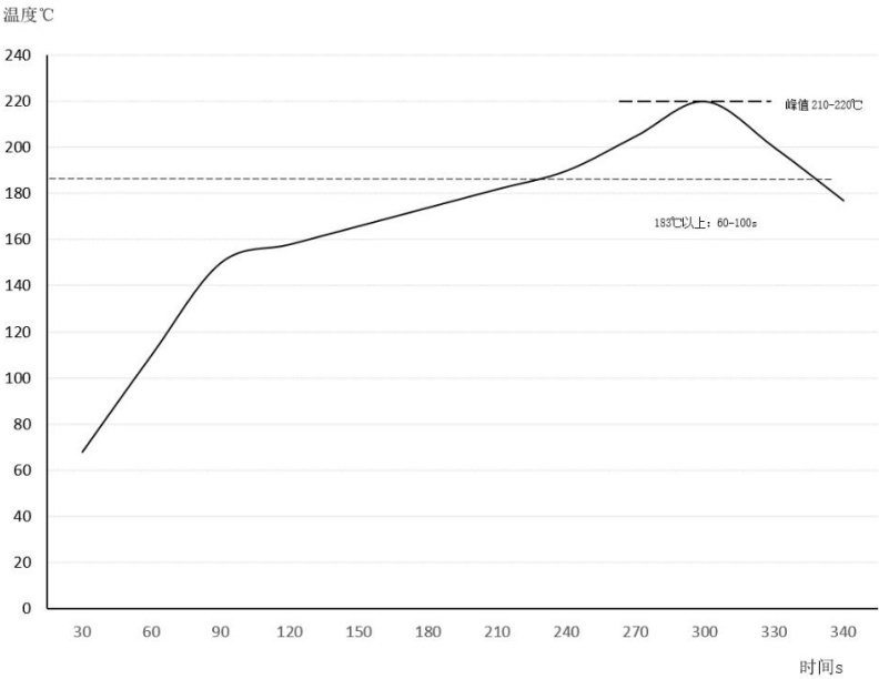
图 11 建议的回流焊曲线
