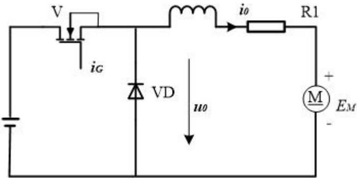
图 9 典型开关电路
