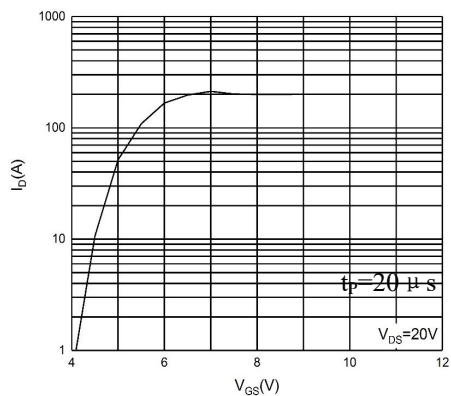
图 1 转移特性曲线
