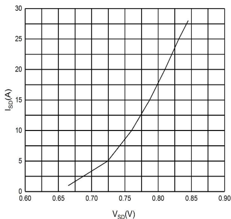
图 2 体二极管特性曲线
