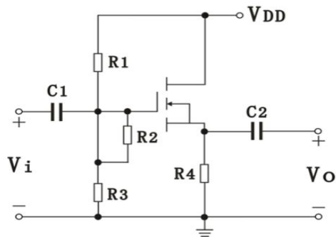
图 10 共漏极放大电路
