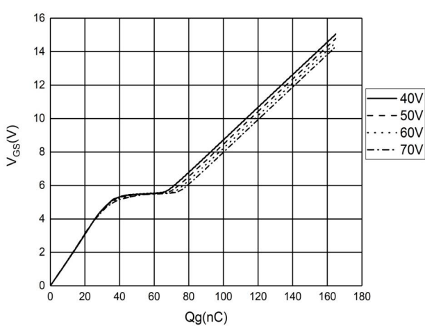
图 5 V_{GS}-Q_g 特性曲线
