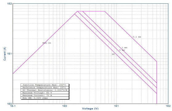
图 6 安全工作区曲线
