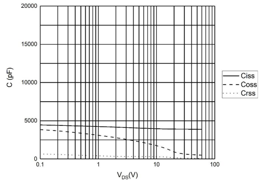
图 4 电容曲线
