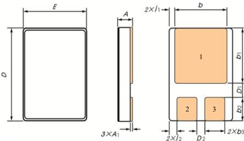
图 7 T0-257 外形尺寸
