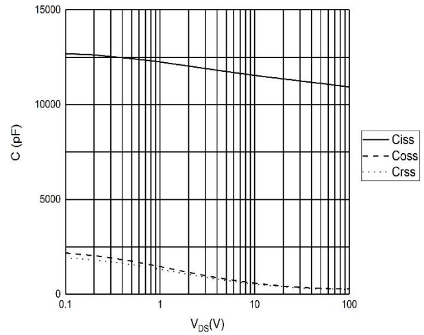
图 4 电容曲线
