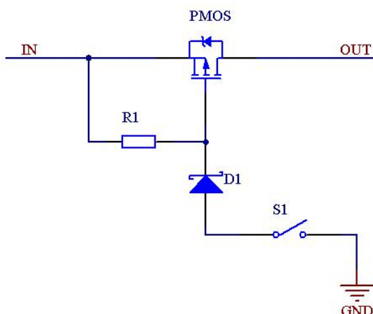
图 9 典型开关电路
