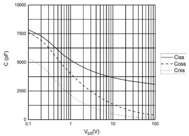
图 4 电容曲线
