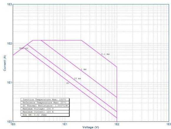
图 6 安全工作区曲线 8 外形尺寸
