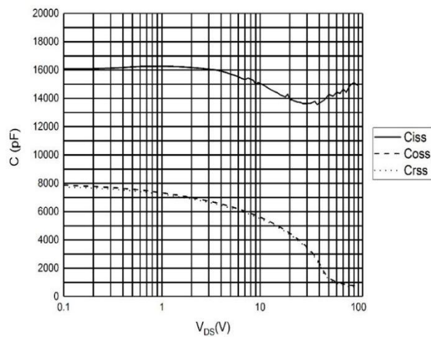
图 4 电容曲线
