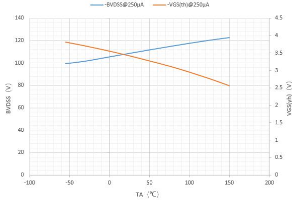
图 2 漏源击穿电压、阈值电压特性曲线
