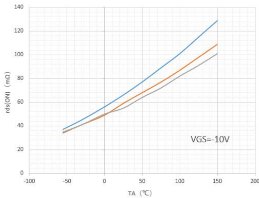
图 1 导通电阻特性曲线
