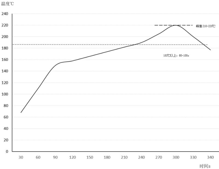
图 8 建议的回流焊曲线
