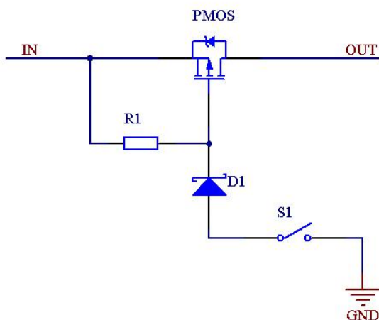
图 7 典型开关电路
