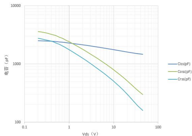
图4 电容特性曲线
