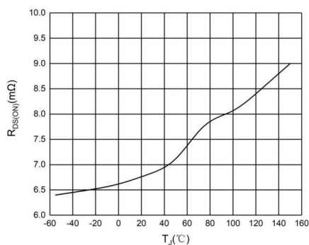
图 3 R_{DS(on)}-T_A 特性曲线
