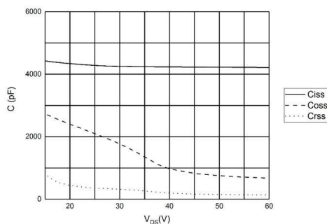
图 4 电容曲线
