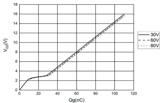
图 5 V_{GS}-Q_g 特性曲线
