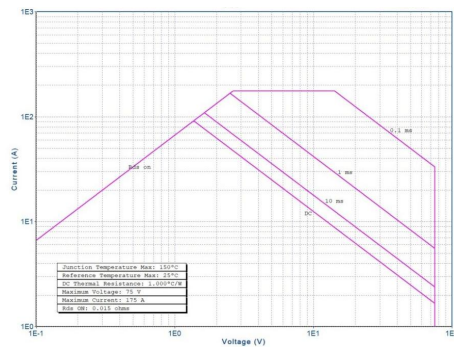
图 6 安全工作区曲线
