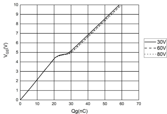
图 5 V_{GS} - Q_g 特性曲线
