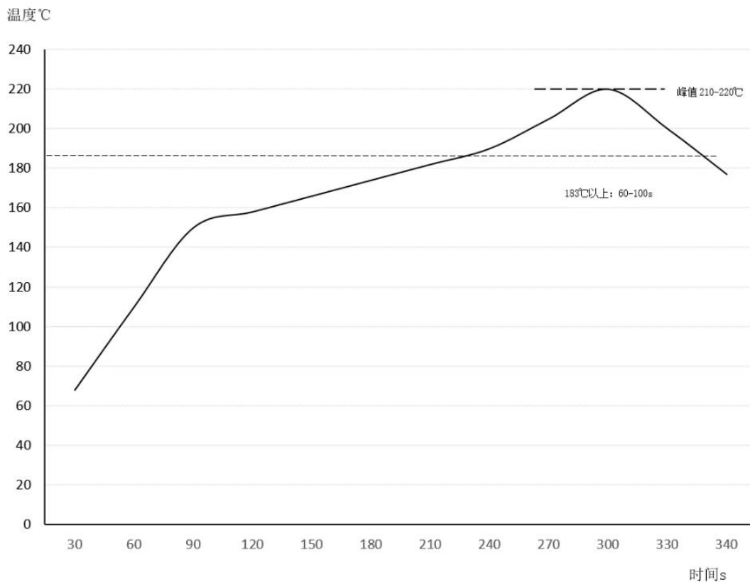
图 11 建议的回流焊曲线
