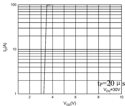
图 1 转移特性曲线
