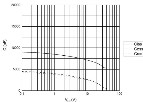
图 4 电容曲线
