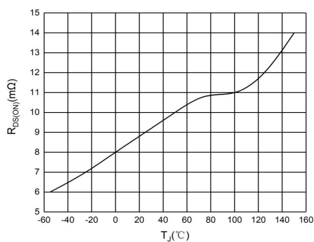
图 3 R_{DS(on)} - T_J 特性曲线
