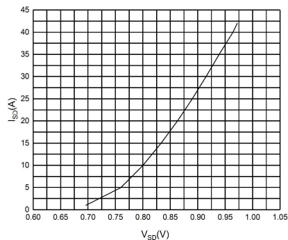
图 2 体二极管特性曲线
