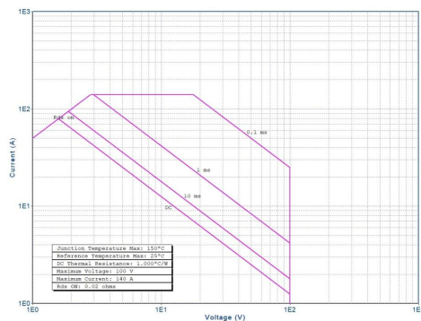
图 6 安全工作区曲线
