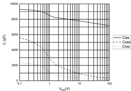
图 4 电容曲线
