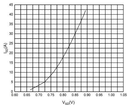
图 2 体二极管特性曲
