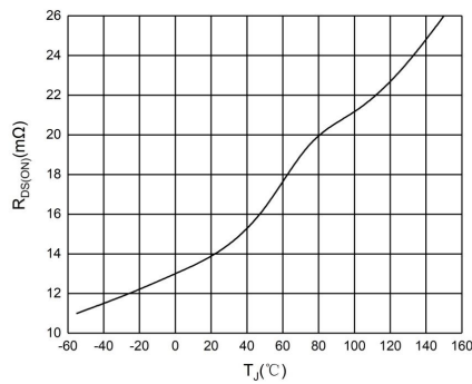
图 3 R_{DS(on)} - T_J 特性曲线
