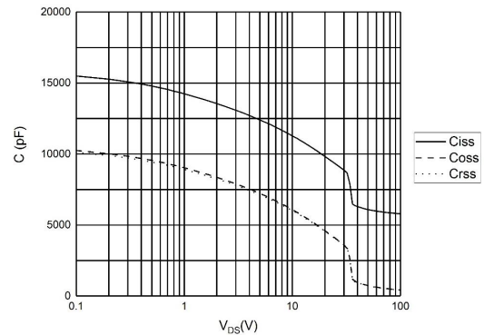
图 4 电容曲线
