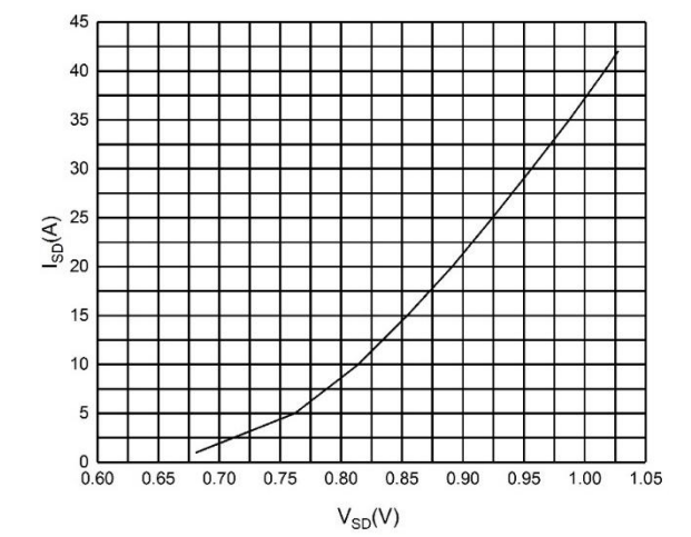
图 2 体二极管特性曲线
