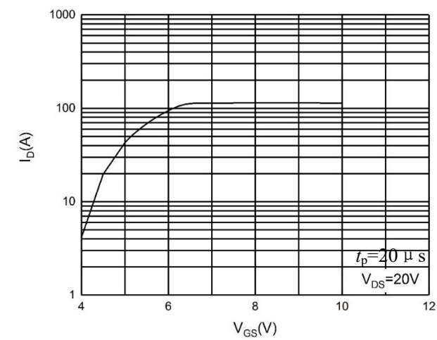
图 1 转移特性曲线
