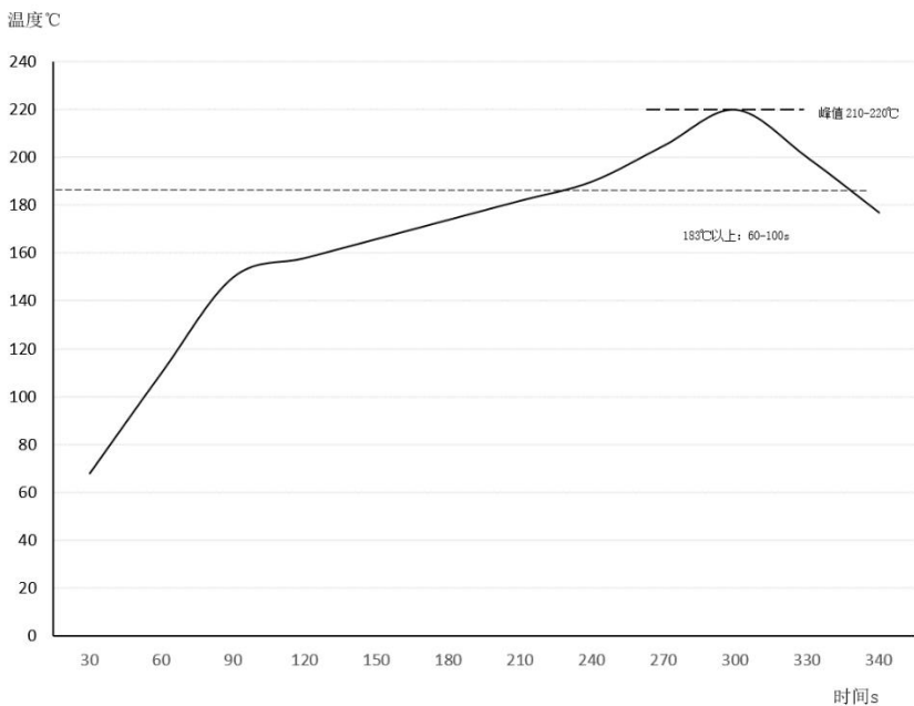
图 11 建议的回流焊曲线
