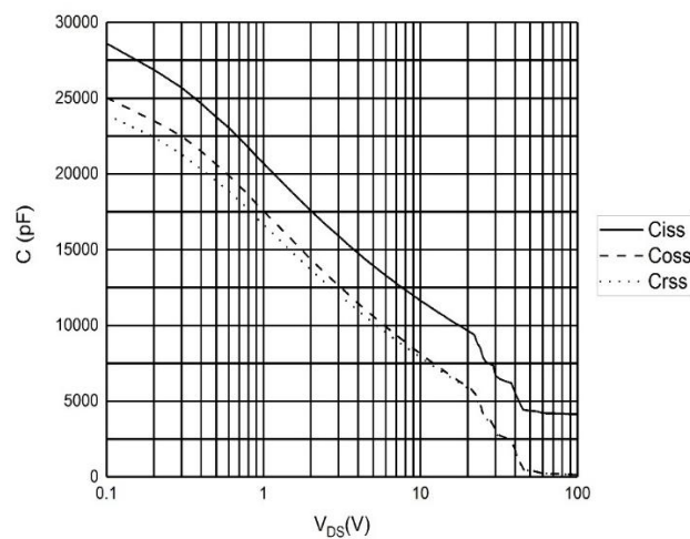
图 4 电容曲线
