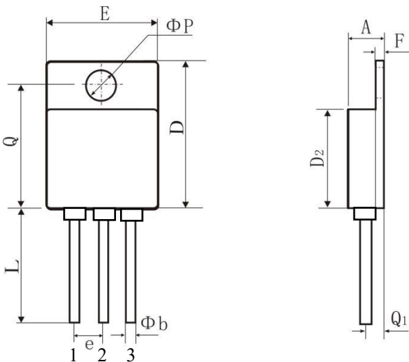
图 7 SMD-1 型封装外形尺寸
