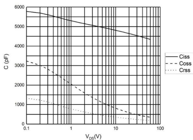
图 4 电容曲线
