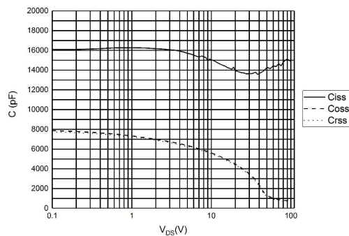
图 4 电容曲线
