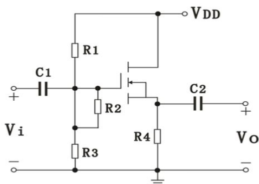
图 9 共漏极放大电路
