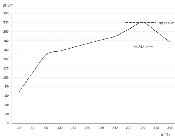
图 10 建议的回流焊曲线
