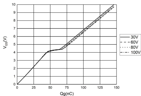
图 5 V_{GS}-Q_g 特性曲线
