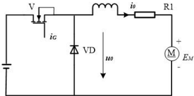
图 8 典型开关电路
