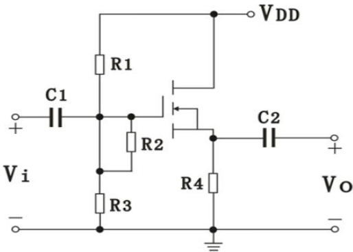
图 7 共漏极放大电路
