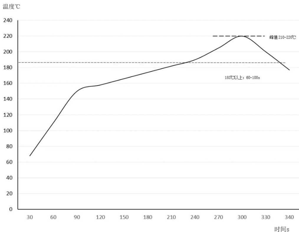
图 8 建议的回流焊曲线
