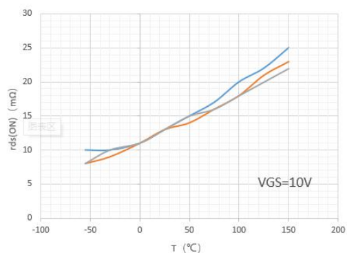
图 1 导通电阻特性曲线
