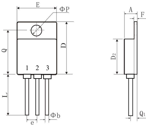
图 4 SMD-0.5、SMD-1 型封装外形尺寸
