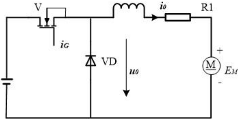
图 6 典型开关电路
