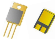
TO-257 型 SMD-0.5 型 TO-254 型 SMD-1 型
