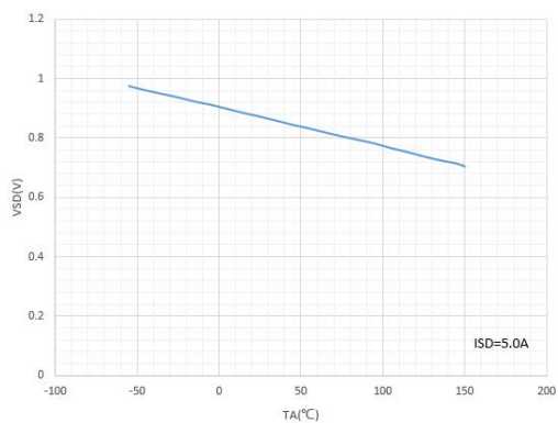
图3 体二极管正向压降特性曲线
