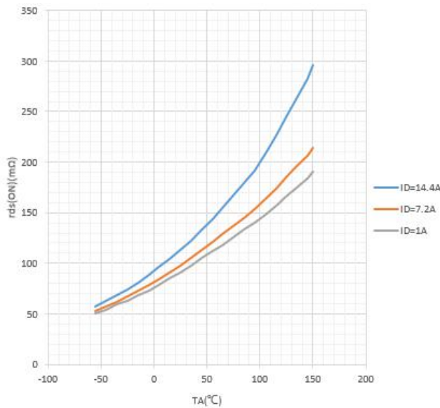
图 1 导通电阻特性曲线
