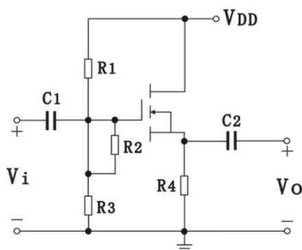
图 8 共漏极放大电路
