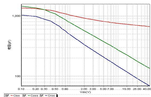
图4 电容特性曲线
