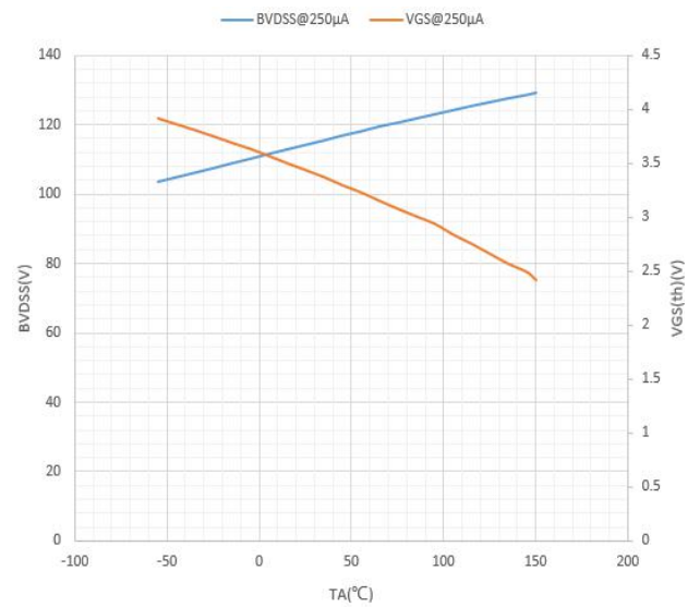
图 2 漏源击穿电压、阈值电压特性曲线
