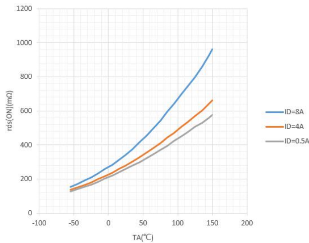
图 1 导通电阻特性曲线
