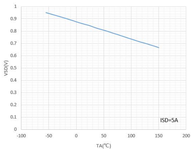
图3 体二极管正向压降特性曲线
