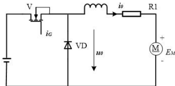
图 7 典型开关电路
