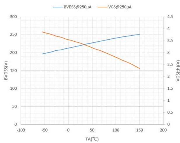
7.2 不同温度下的漏源击穿电压及开启阈值电压曲线
