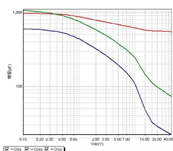
图4 电容特性曲线
