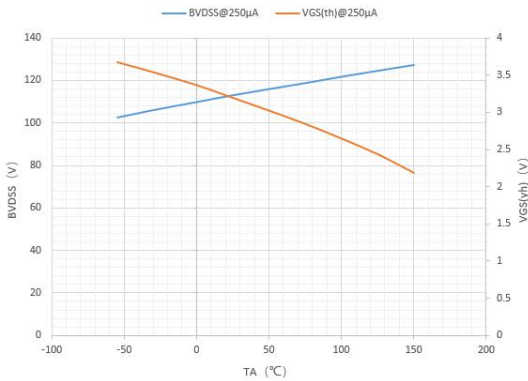
图 2 漏源击穿电压、阈值电压特性曲线
