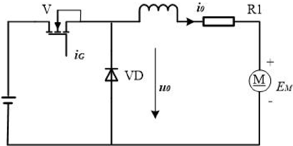
图 6 典型开关电路
