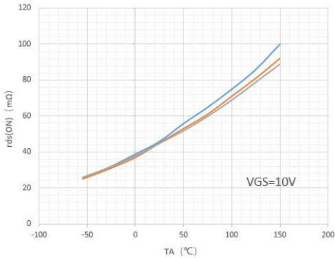
图 1 导通电阻特性曲线
