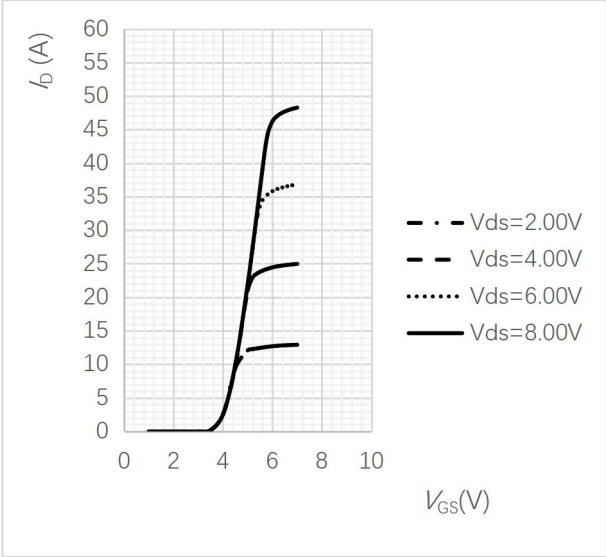
图 2 转移曲线
