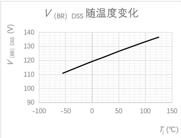
图9 漏源击穿电压随温度变化曲线
