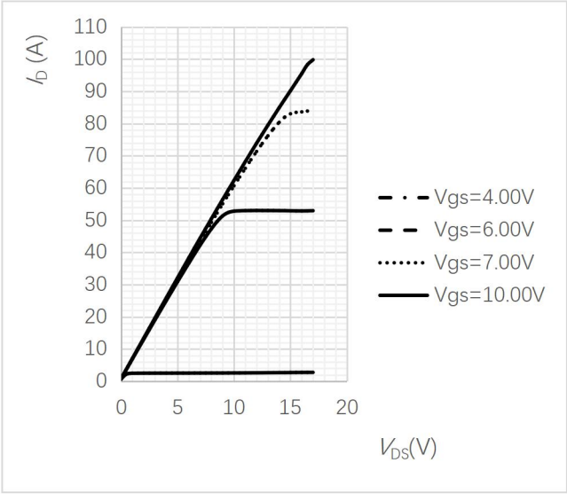
图 1 输出曲线
