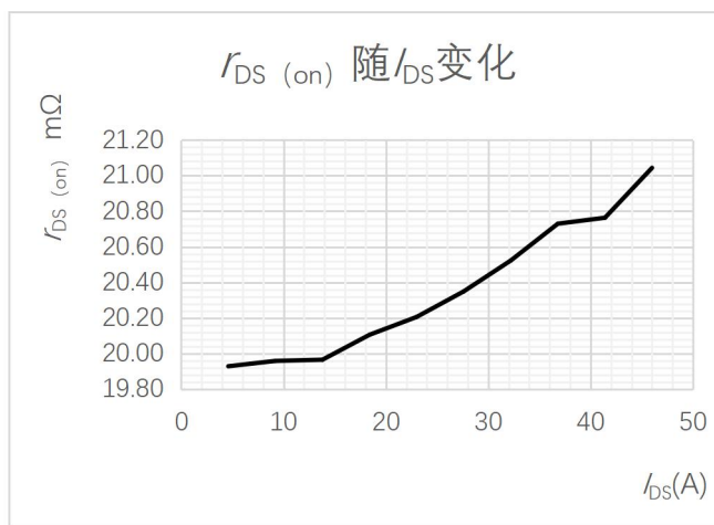
图 7 导通电阻随电流变化曲线
