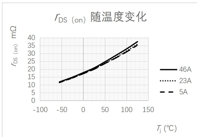
图 5 导通电阻随温度变化曲线
