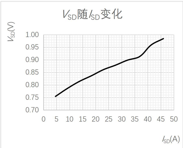
图10 体二极管正向压降曲线
