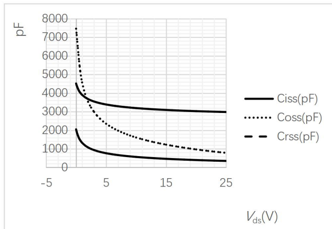
图 3 电容对电压变化曲线
