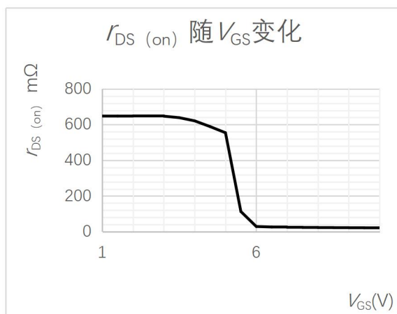
图 6 导通电阻随开启电压变化曲线
