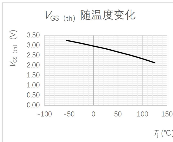
图 8 开启电压随温度变化曲线
