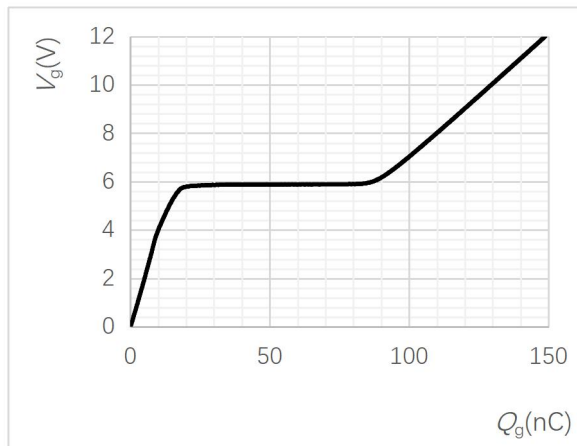
图 4 栅电荷曲线
