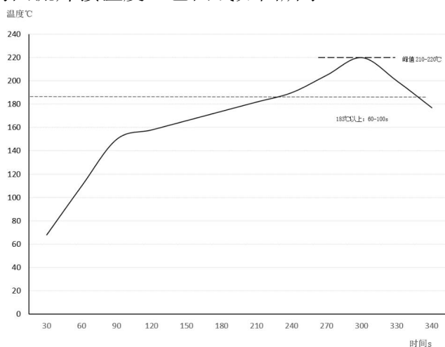
图 13 建议的回流焊曲线
