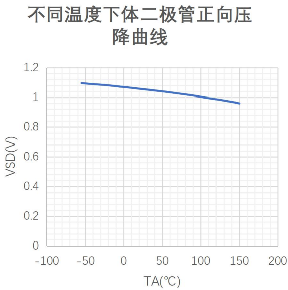
图3 体二极管正向压降特性曲线
