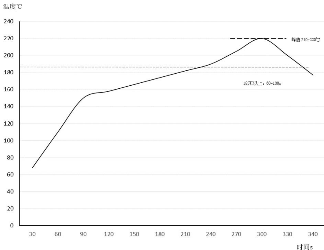
图 8 建议的回流焊曲线
