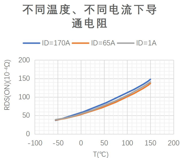
图 1 导通电阻特性曲线
