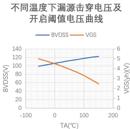
图 2 漏源击穿电压、阈值电压特性曲线
