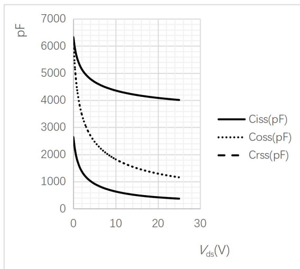
图 3 电容对电压变化曲线
