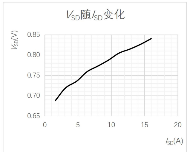
图 8 体二极管正向压降曲线 ( I_b=16A )
