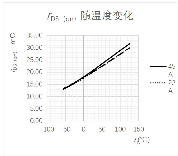
图 4 导通电阻随温度变化曲线
