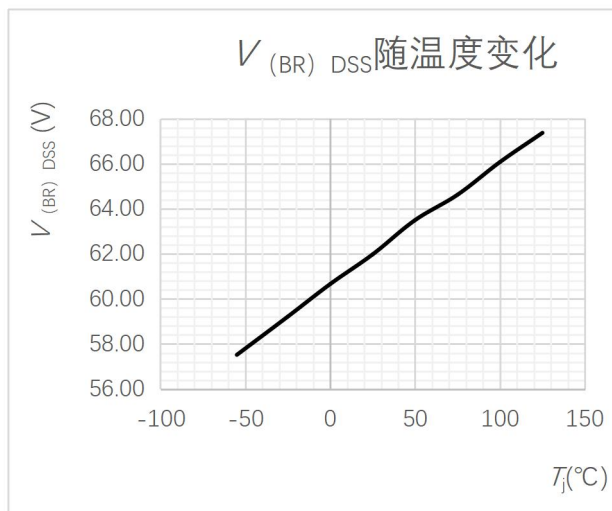
图 7 漏源击穿电压随温度变化曲线
