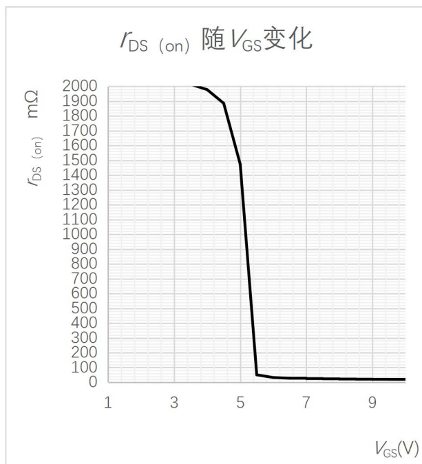
图 5 导通电阻随开启电压变化曲线 ( I_D=16A )
