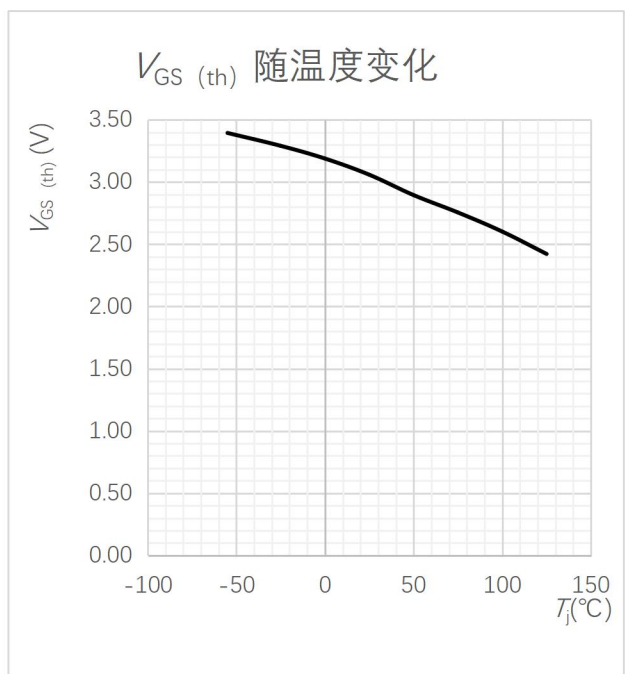
图 6 开启电压随温度变化曲线
