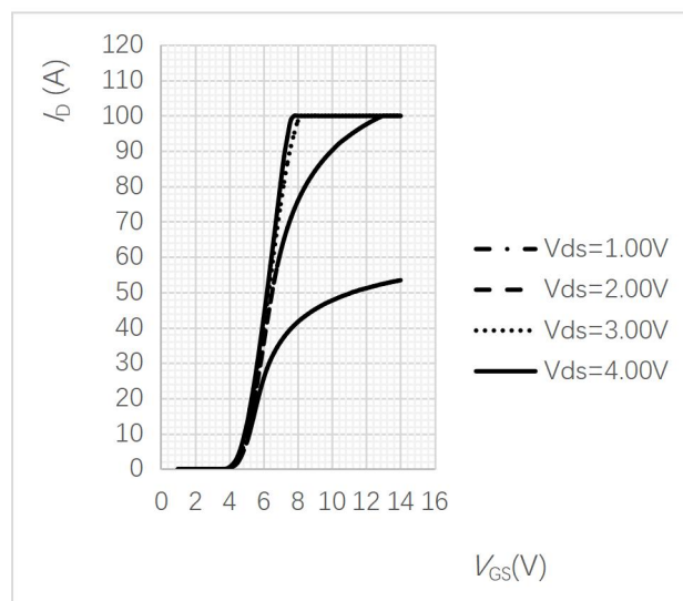
图 2 转移曲线
