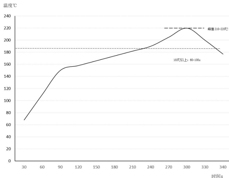
图 4 建议的回流焊曲线
