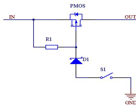
图 3 典型开关电路
