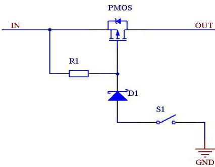
图 13 典型开关电路
