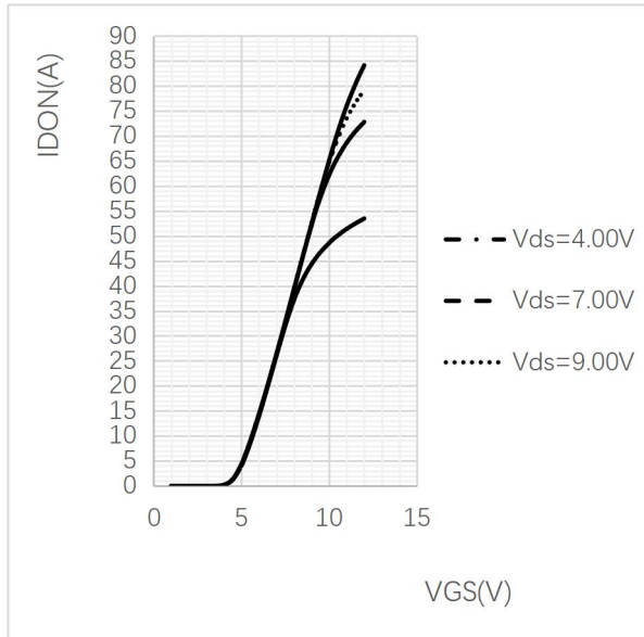
图 2 LYPM5305G 转移曲线
