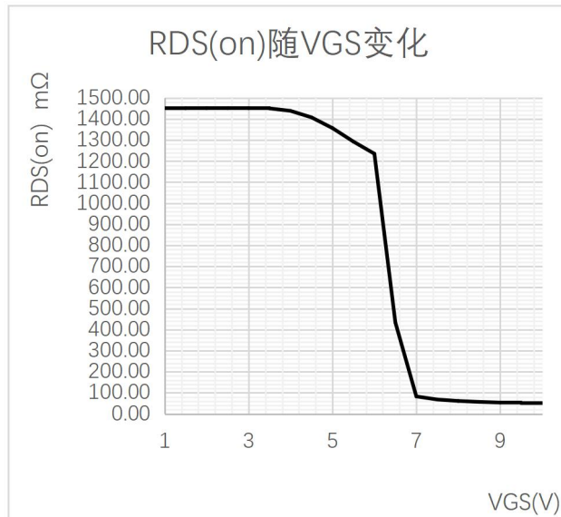
图 6 LYPM5305G 导通电阻随开启电压变化曲线
