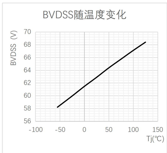
图 9 LYPM5305G 漏源击穿电压随温度变化曲线
