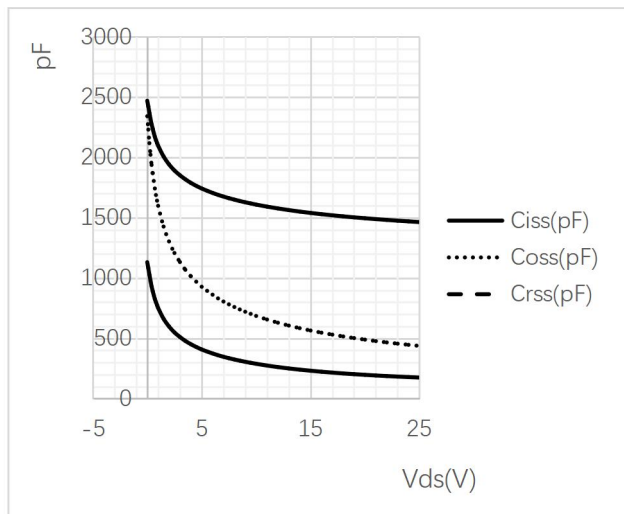
图 3 LYPM5305G 电容对电压变化曲线
