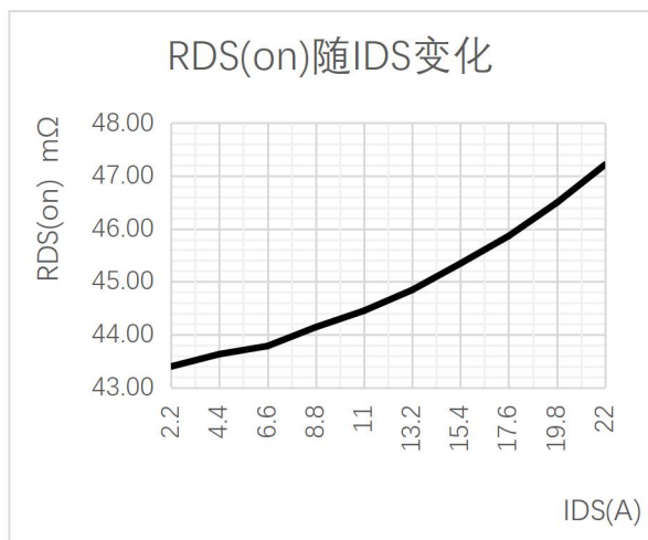
图 7 LYPM5305G 导通电阻随电流变化曲线
