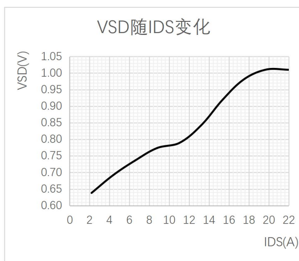
图 10 LYPM5305G 体二极管正向压降曲线
