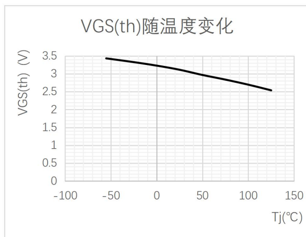
图 8 LYPM5305G 开启电压随温度变化曲线
