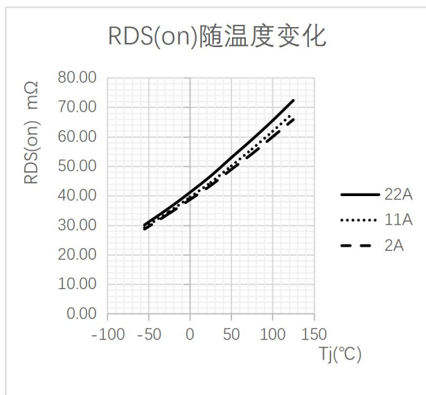
图 5 LYPM5305G 导通电阻随温度变化曲线
