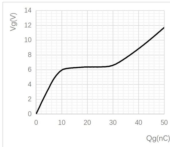
图 4 LYPM5305G 栅电荷曲线
