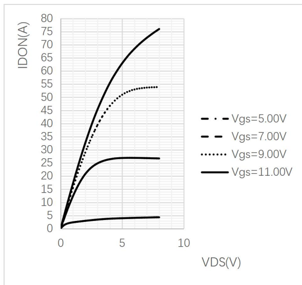
图 1 LYPM5305G 输出曲线
