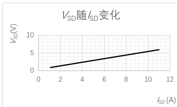
图 8 体二极管正向压降曲线
