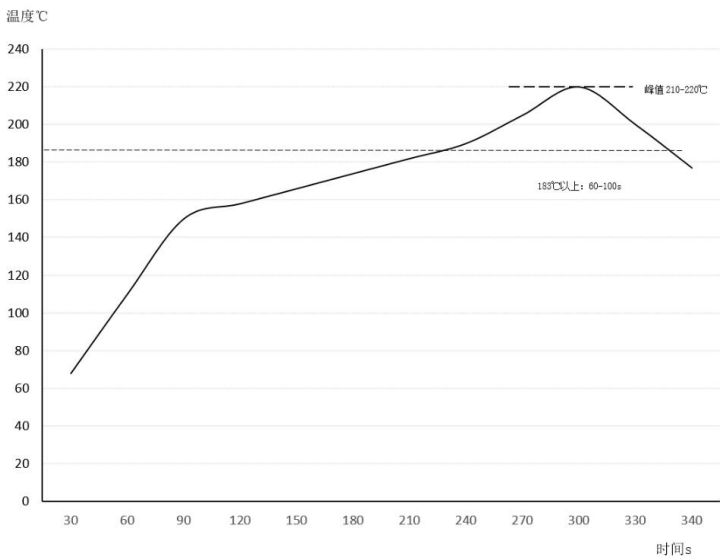
图 12 建议的回流焊曲线
