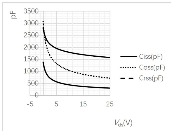
图 3 电容对电压变化曲线
