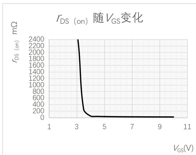
图 6 导通电阻随开启电压变化曲线
