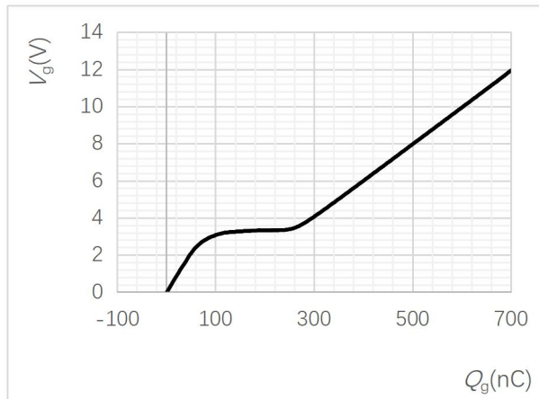
图 4 栅电荷曲线
