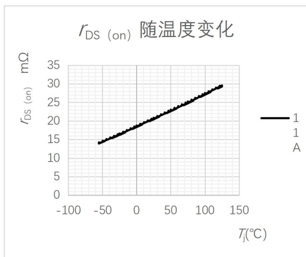
图 5 导通电阻随温度变化曲线
