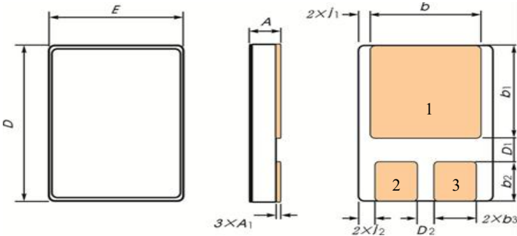
图 9 T0-257 外形尺寸
