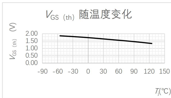
图 7 开启电压随温度变化曲线
