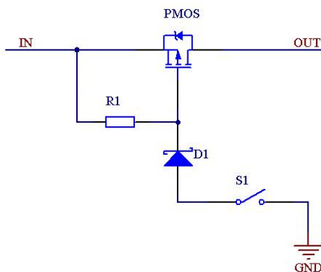
图 11 典型开关电路
