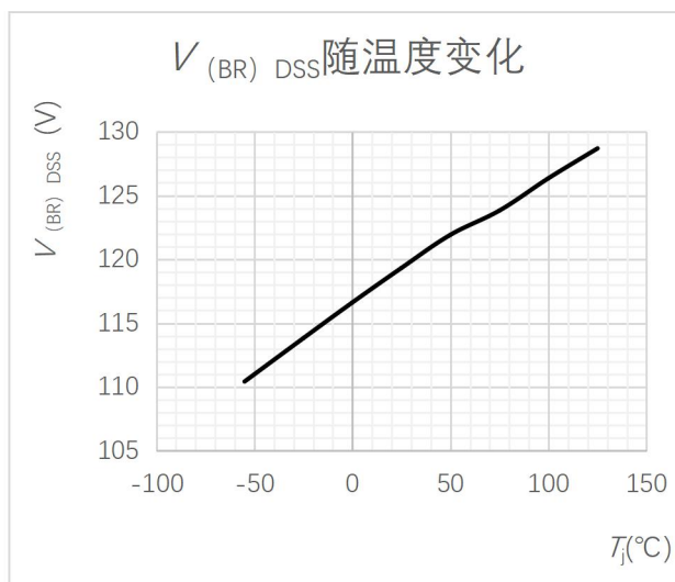
图 9 漏源击穿电压随温度变化曲线
