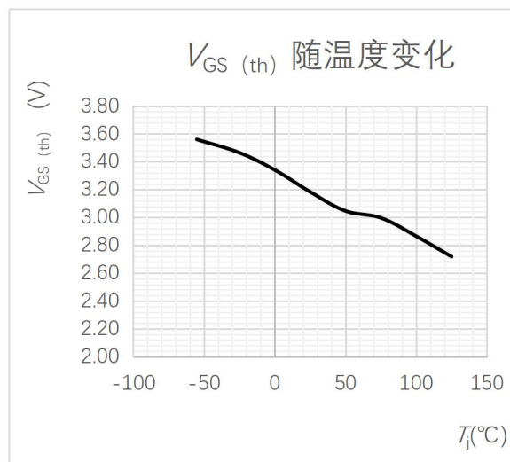
图 8 开启电压随温度变化曲线
