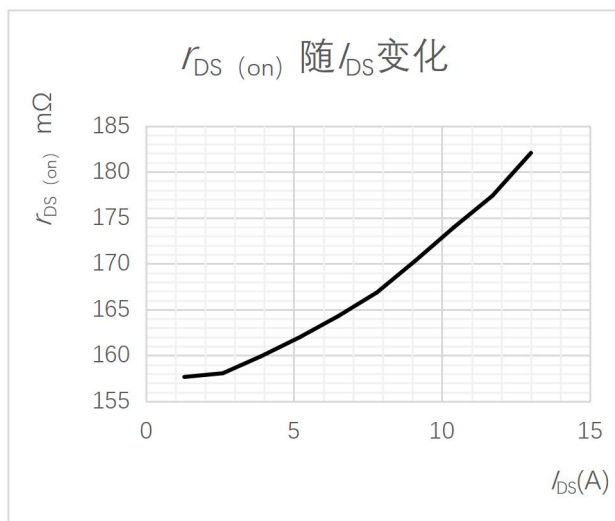
图 7 导通电阻随电流变化曲线
