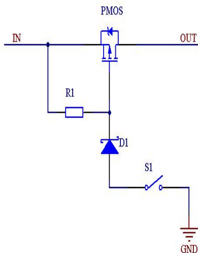
图 13 典型开关电路
