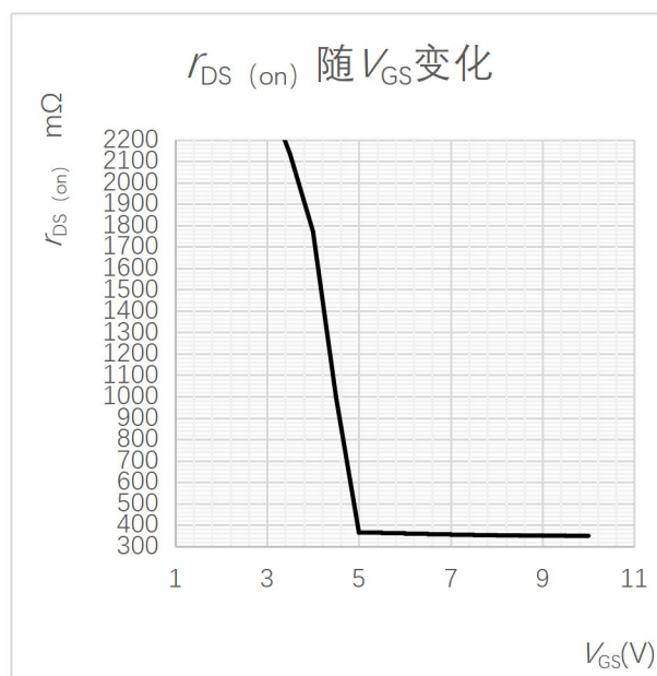
图 6 导通电阻随开启电压变化曲线
