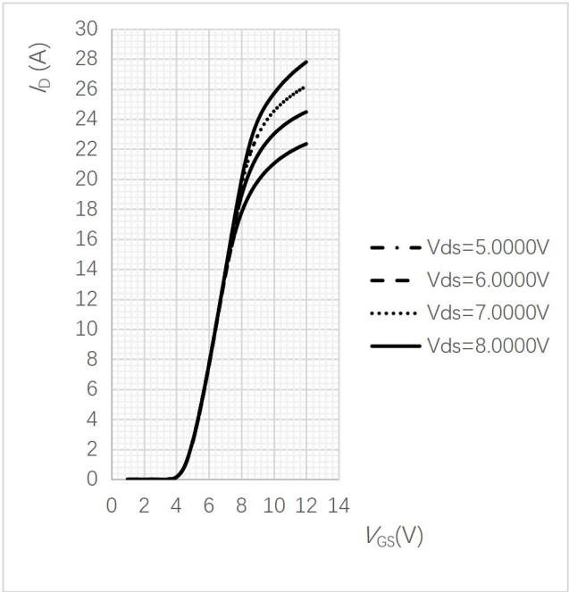
图 1 输出曲线
