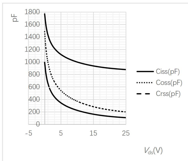
图 3 电容对电压变化曲线
