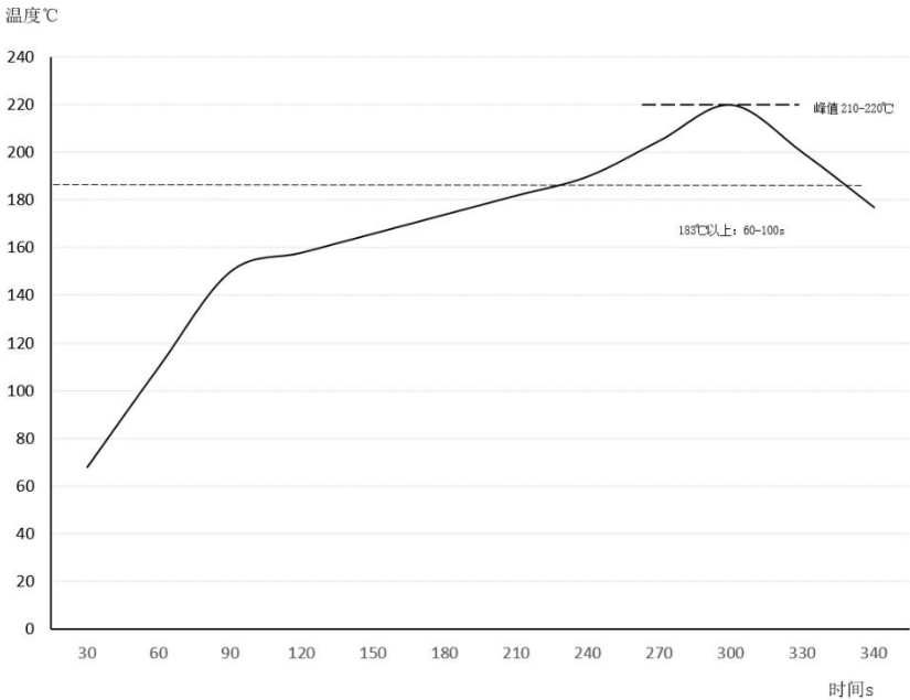
图 14 建议的回流焊曲线
