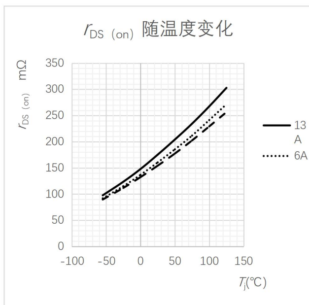
图 5 导通电阻随温度变化曲线
