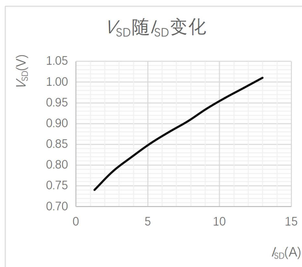
图 10 体二极管正向压降曲线
