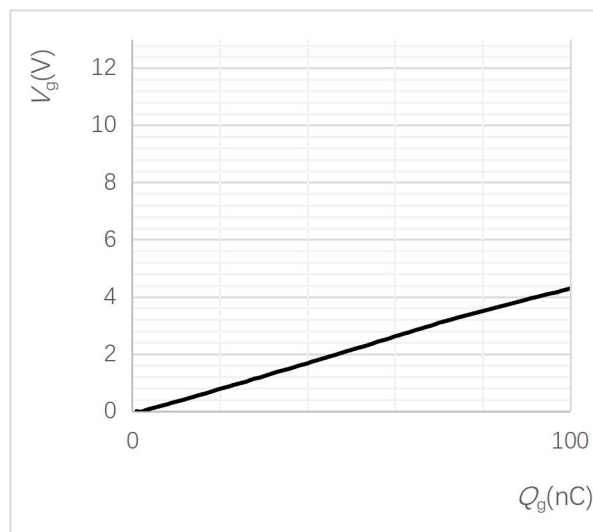
图 4 栅电荷曲线
