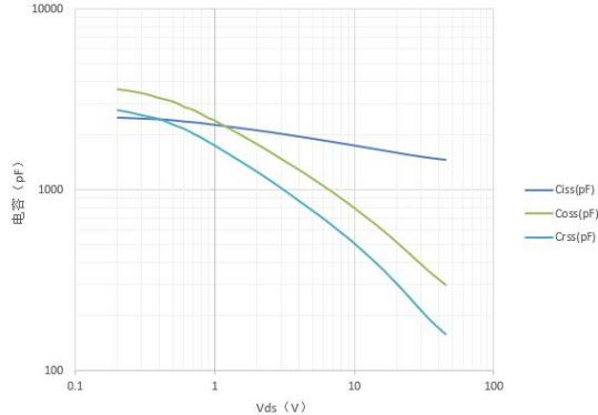
图4 电容特性曲线
