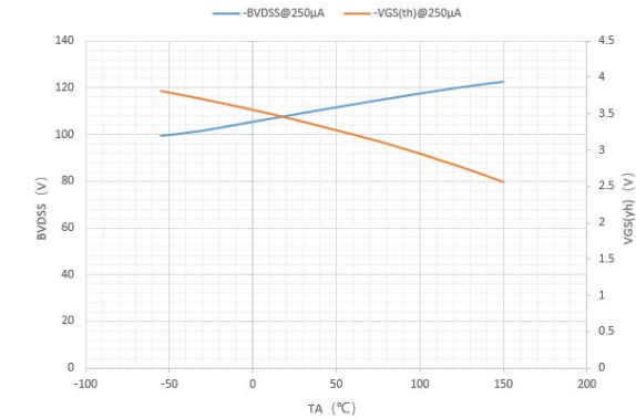
7.2 不同温度下的漏源击穿电压及开启阈值电压曲线
